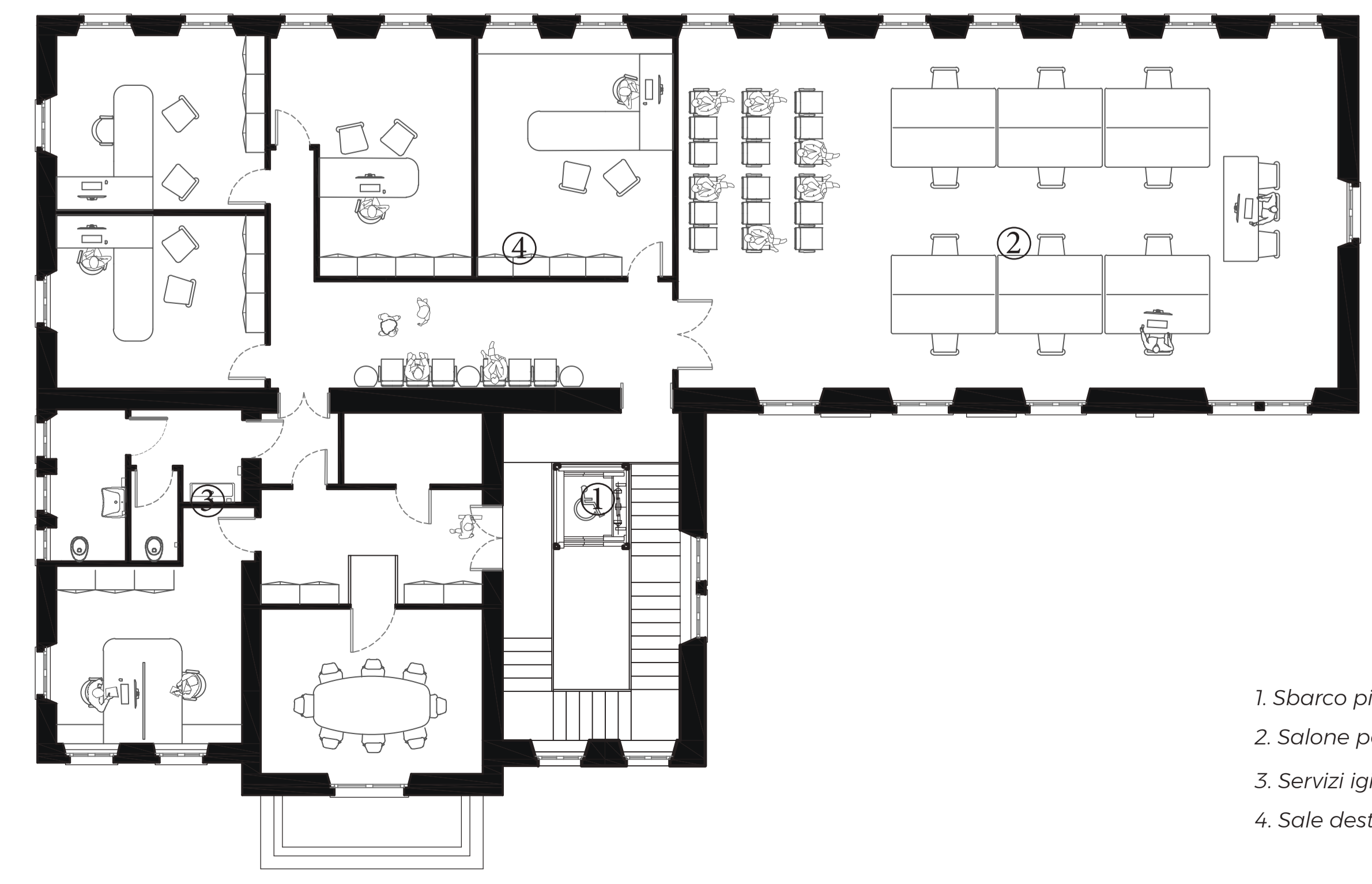
Piano Primo Scala 1:100
